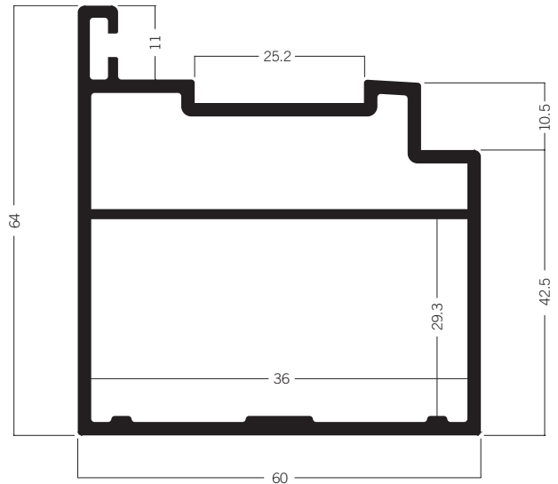
C 302 Door frame extrusion 60 × 64 mm 9.51 kg | 6000 mm
