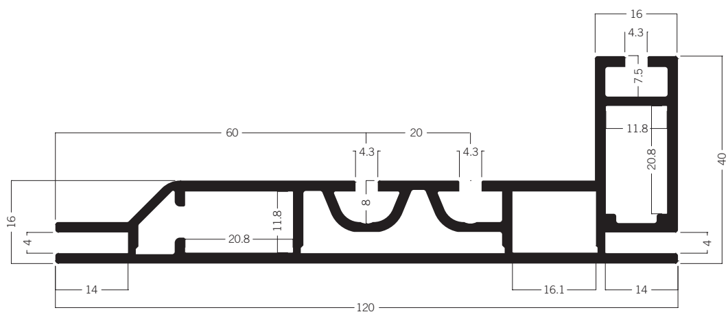
M 1915 Tension fabric extrusion für for light frame 120 mm 11.90 kg | 6000 mm
