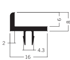
E 442 Supporting edge 0.40 kg | 5000 mm
